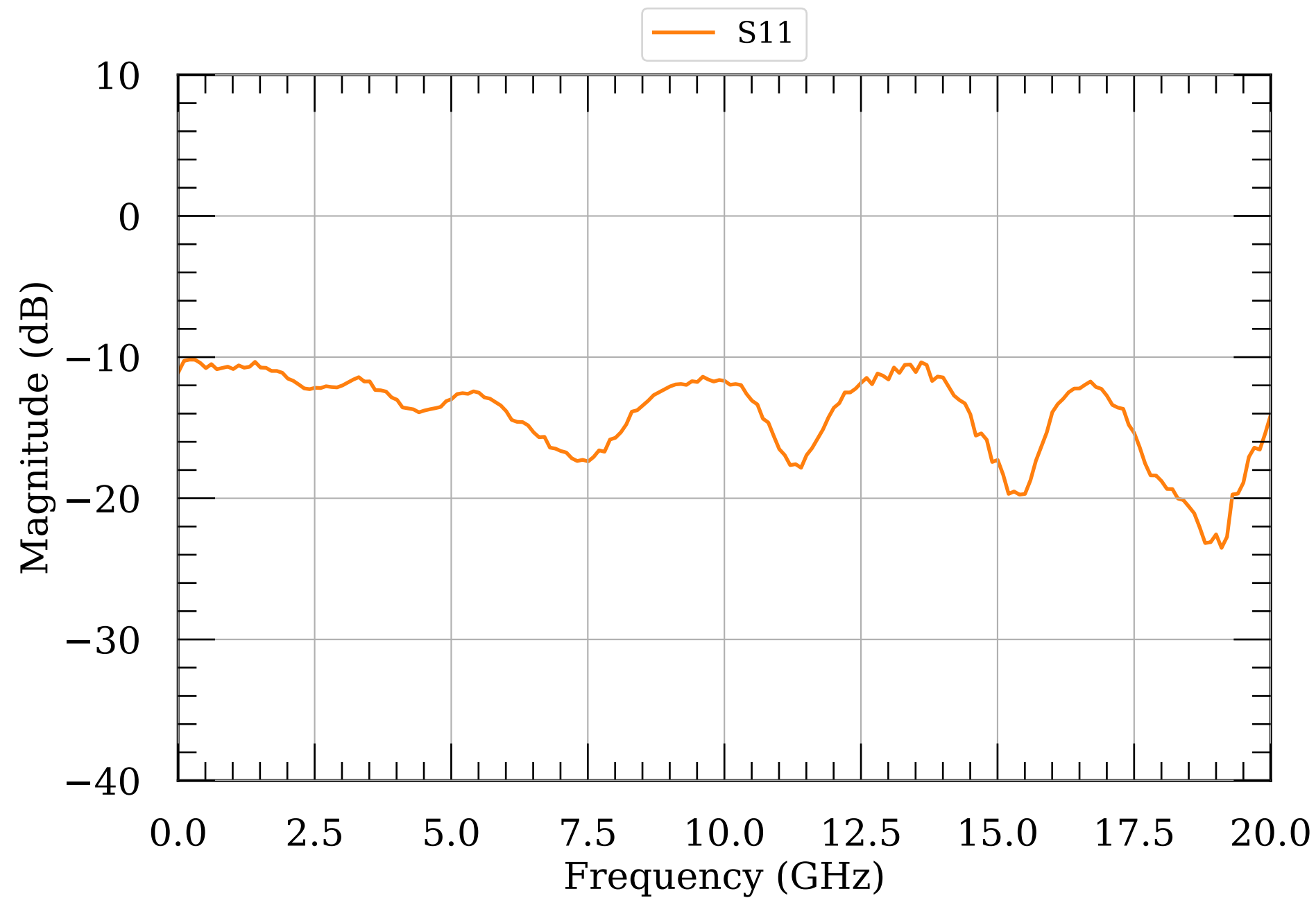
LNA S-params module077
